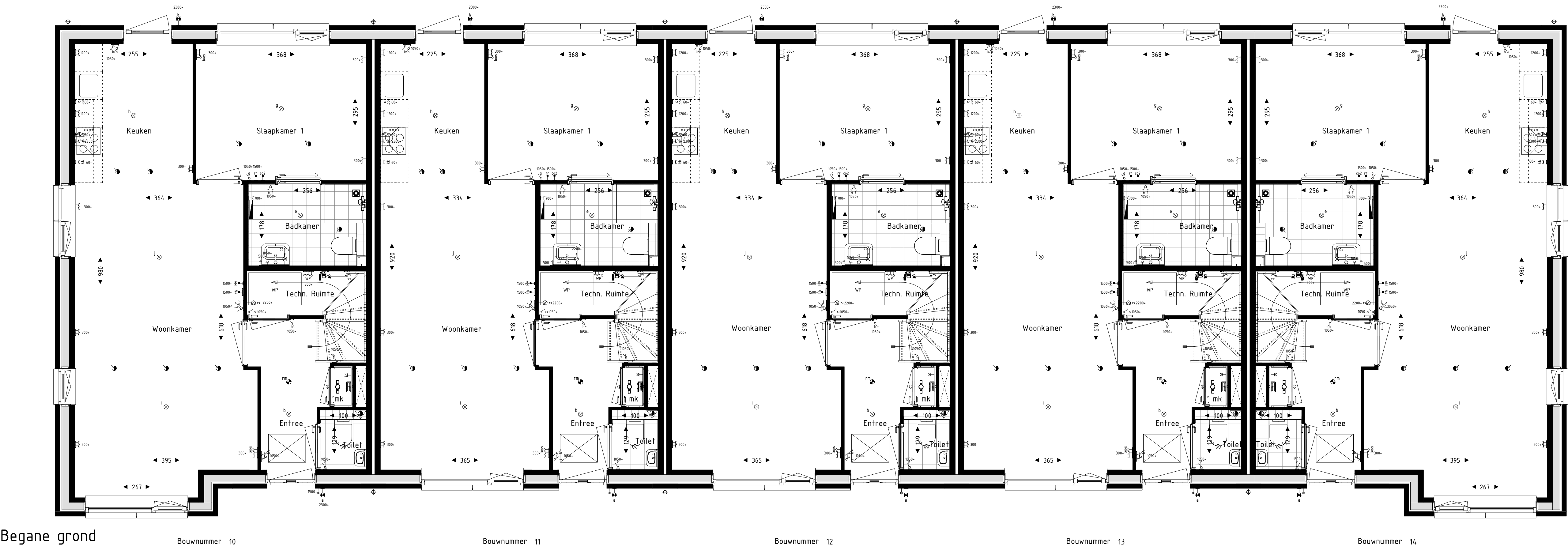
Begane grond
