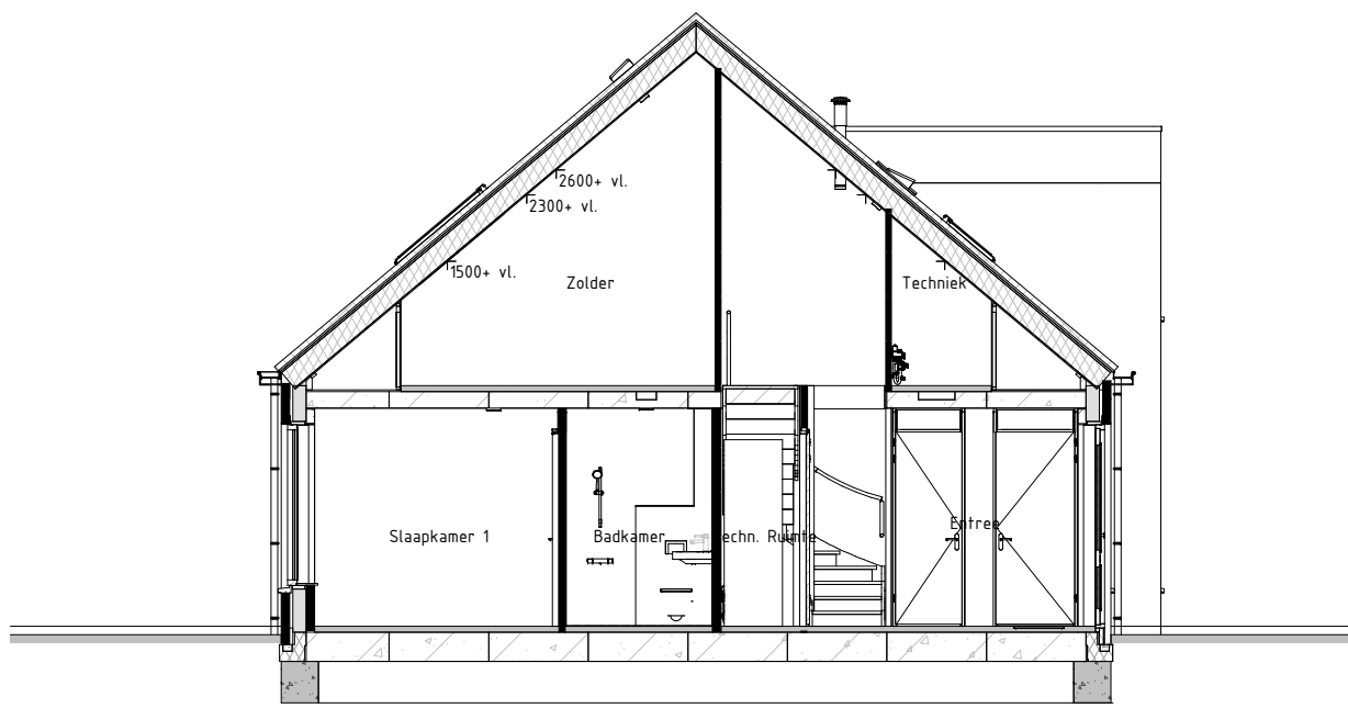
Doorsnede AA
